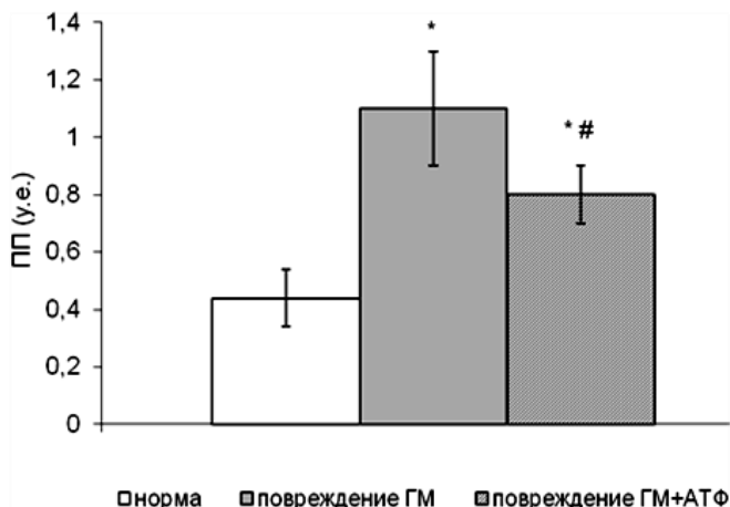
Рис. 1. Изменение значения обобщенного показателя пероксидации (ОПП) у животных контрольной (повреждение) и основной экспериментальной (повреждение + АТФ) групп на 3 сутки после моделирования локального компрессионного повреждения головного мозга. * - P<0,01 , ** - P<0,05 в сравнении с ложнооперированной группой; # - P<0,05 в сравнении с контрольной группой
