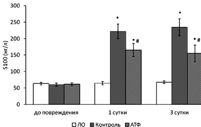
Рис. 2. Концентрация белка S100 (нг/л) в плазме крови при моделировании локального компрессионного повреждения коры головного мозга у крыс
