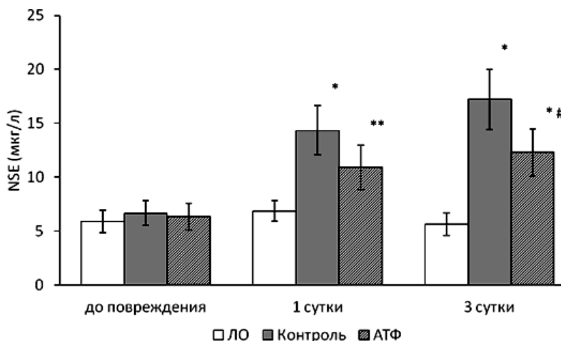
Рис. 1. Концентрация нейроспецифической енолазы (NSE, мкг/л) в плазме крови при моделировании локального компрессионного повреждения коры головного мозга у крыс: «ЛО» – 1 группа (ложнооперированная серия); «Контроль» – 2 группа (контрольная - повреждение головного мозга); «АТФ» – 3 группа (основная, повреждение головного мозга на фоне в/б введения АТФ 50 мг/кг). * - P < 0,01 ** - P < 0,05 в сравнении с исходным уровнем (до повреждения) и 1 группой (ложнооперированная серия); # - P < 0,05 в сравнении со 2 группой (контрольная серия)
