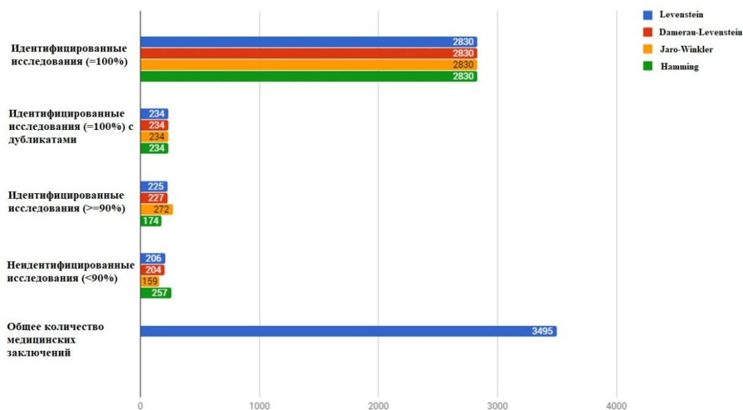
Рис. 3. Сравнительный график результатов работы алгоритмов при использовании букв русского алфавита
