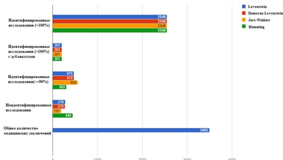
Рис. 2. Сравнительный график результатов работы алгоритмов при использовании букв латинского алфавита
