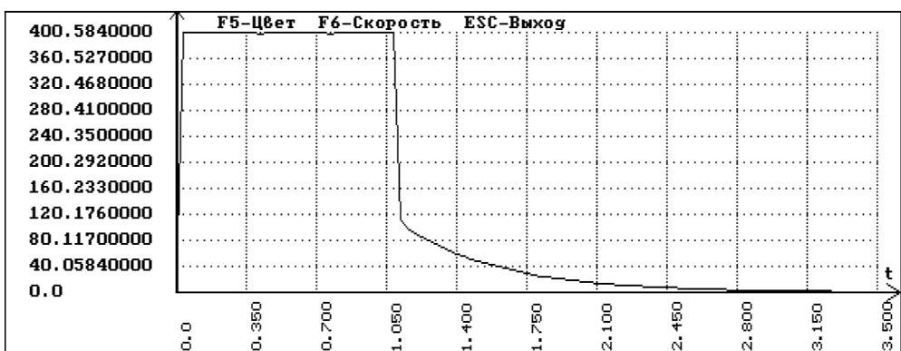
Рис. 2. Переходные процессы при A_3=10000 дискрет
