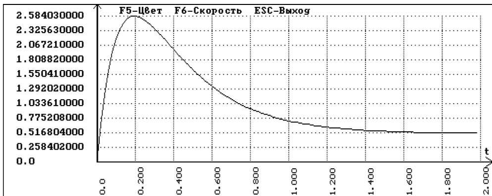
Рис. 1. Переходные процессы в контуре положения при A_1=20 дискрет
