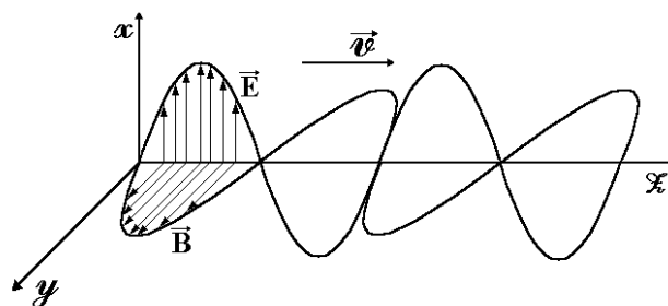
Рис. 3. Движение энергии ЭМВ
